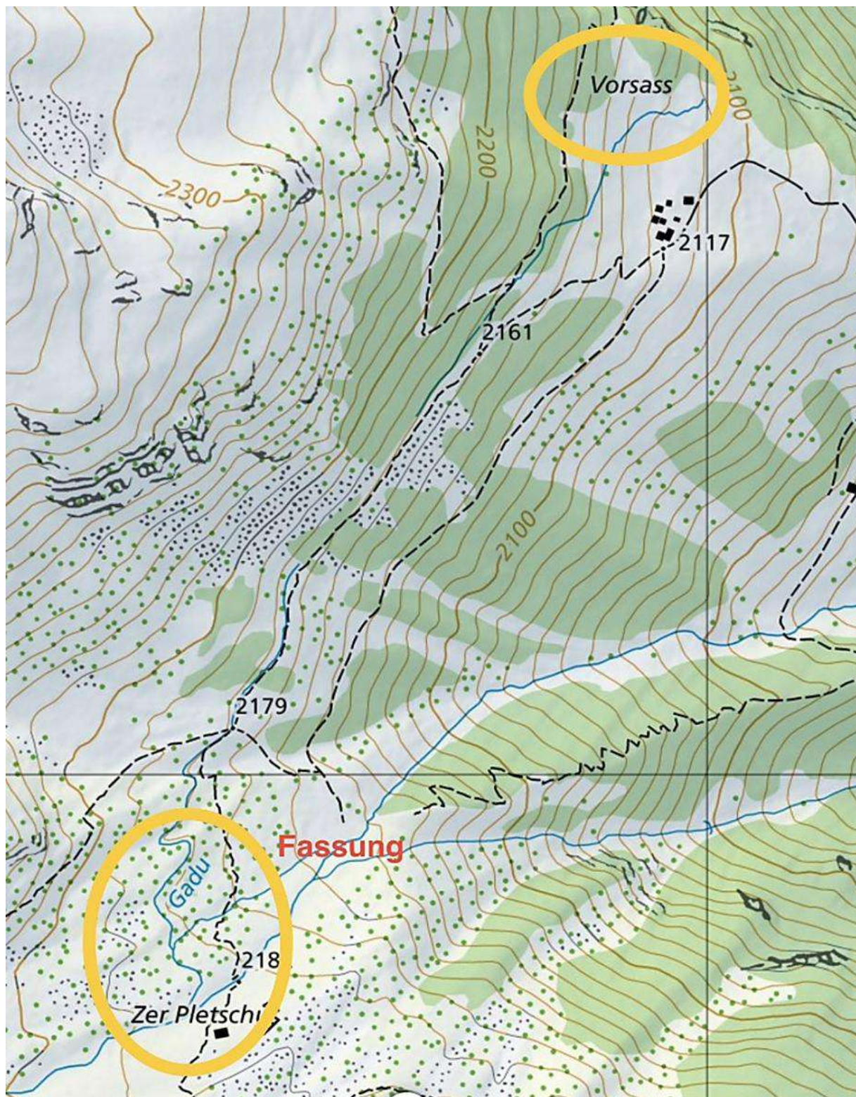
Fassung der Gadu am Vorder Borterbach, oberhalb der Fassung der Spunnu
