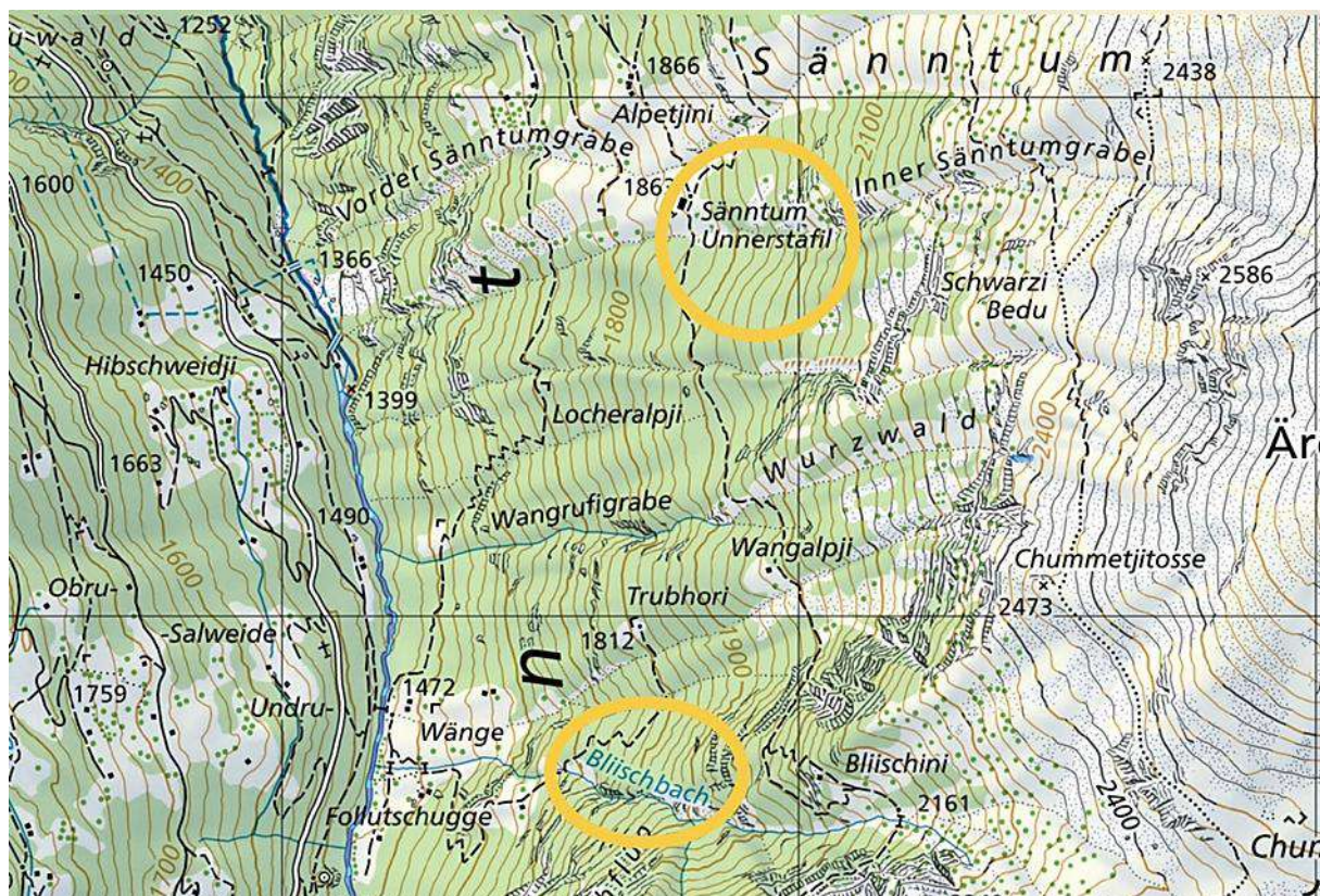
Fassung am Blieschbach, rechtsufrig der Turtmäna, auf der Höhe des Follutschugge
