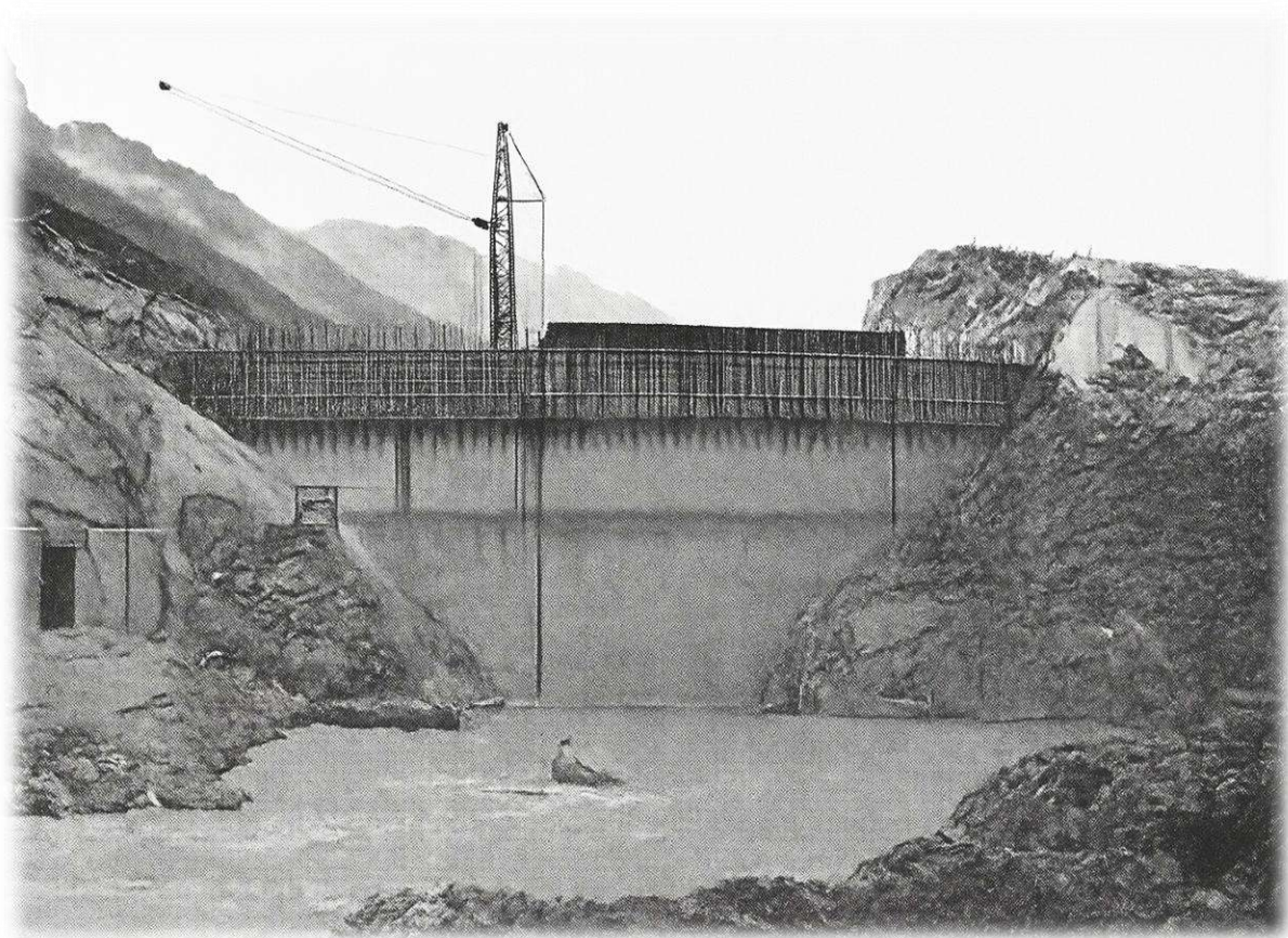
Staumauer Turtmantal : Bauzustand Sommer 1958 (Photo Brügger, Zürich)
