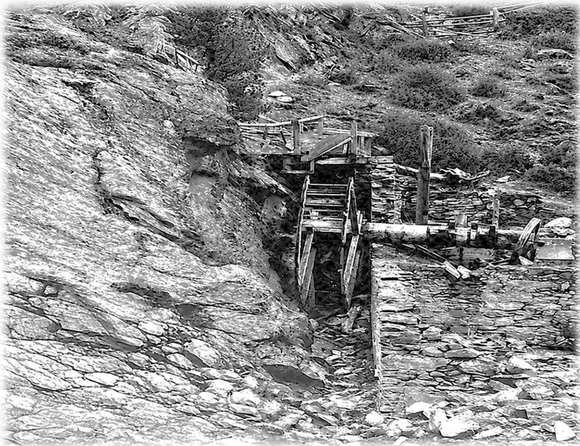
Aufnahme des ca. 3-4 m durchmessenden, überschäftigen Wasserrads. Gut zu erkennen, rechts die Zapfen zur Anhebung der Pochstempel und ganz rechts das Antriebsrad der Transmission.
